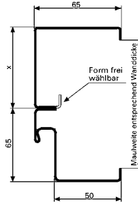
Eckzarge mit Gegenzarge
